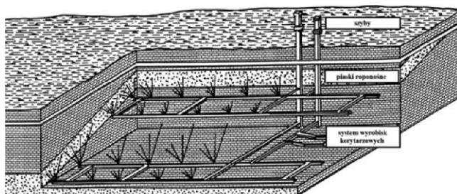
Rys. 9. Koncepcja eksploatacji złoża ropy naftowej z udostępnieniem złoża szybami i rozcinką wyrobiskami górnictwa oraz wykorzystaniem gęstej sieci podziemnych wierceń wg [2]
