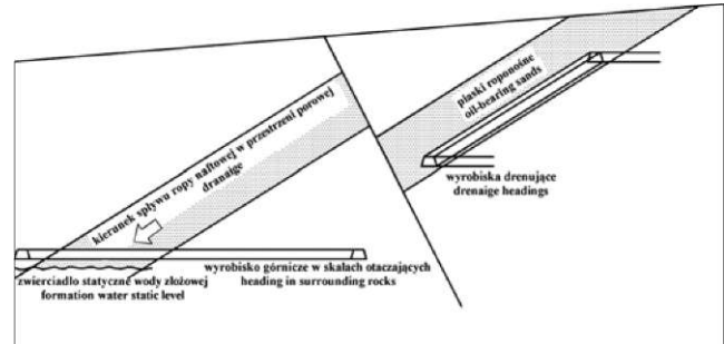
Rys. 5. Schemat drenażu utworów roponośnych wg [3]
